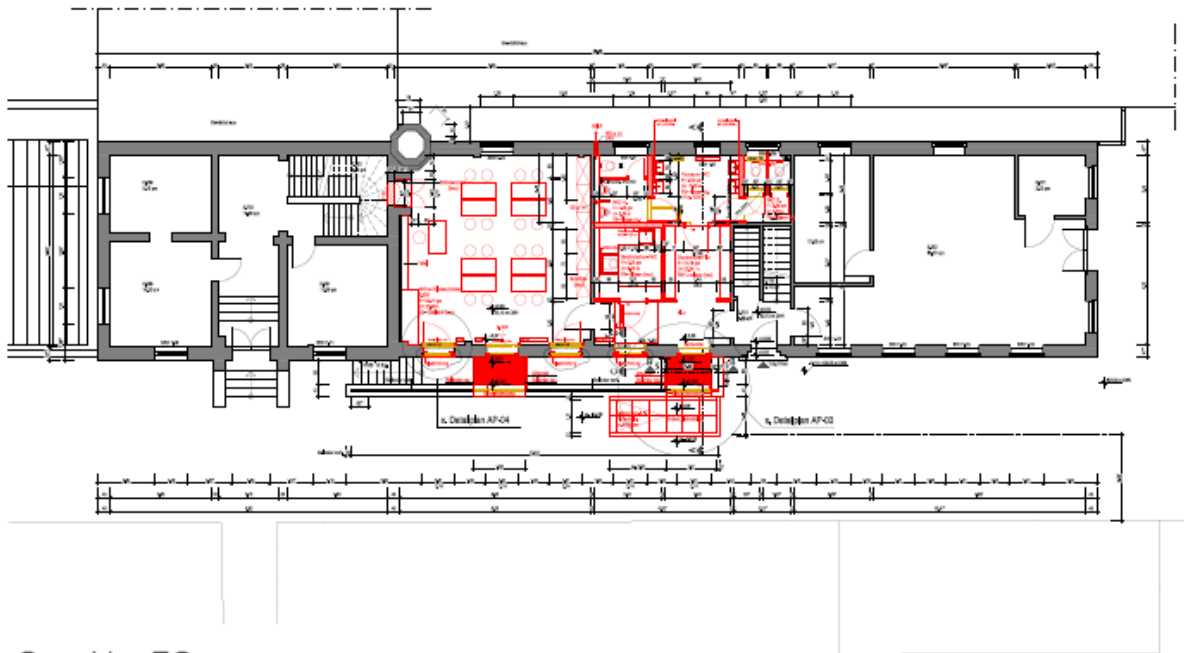
Grundriss EG
